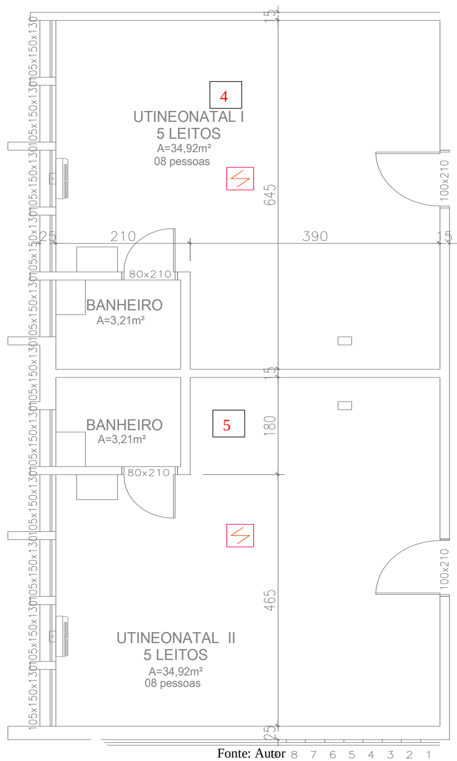
Figura 21- – Planta Baixa do ambientes de UTI Neonatal com pontos de medição.
