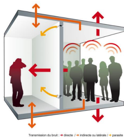
Figura 2- Formas de propagação do som recintos
