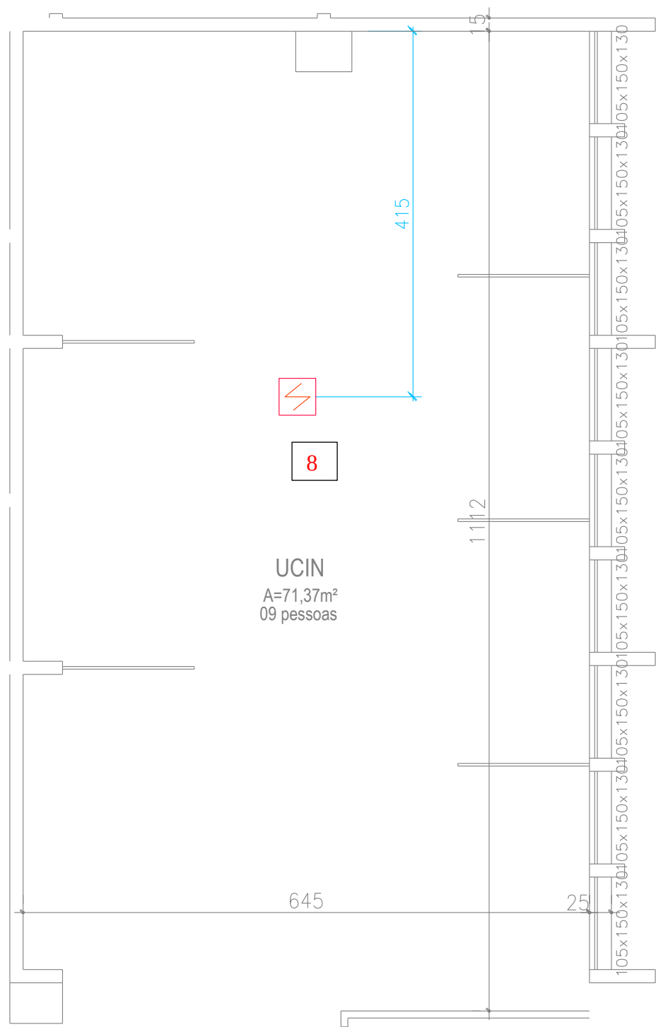
Figura 25- – Planta Baixa do ambientes UCIN com ponto de medição
