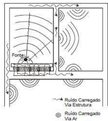
Figura 7- Transmissão de ruído
