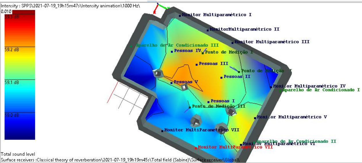
Figura 34 – Simulação do ambiente de Unidade de Terapia Intensiva Pediátrica
