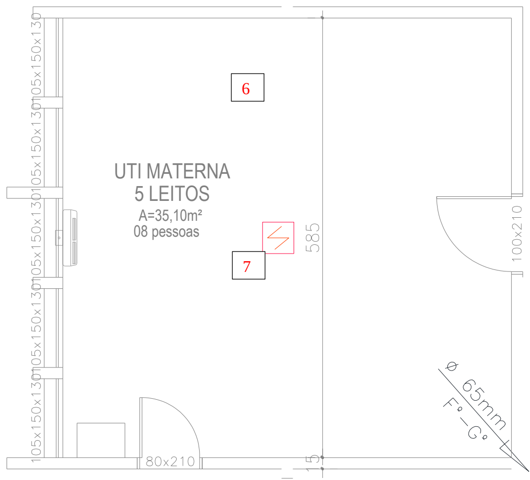
Figura 23- Planta Baixa do ambientes de UTI Materna com pontos de medição.
