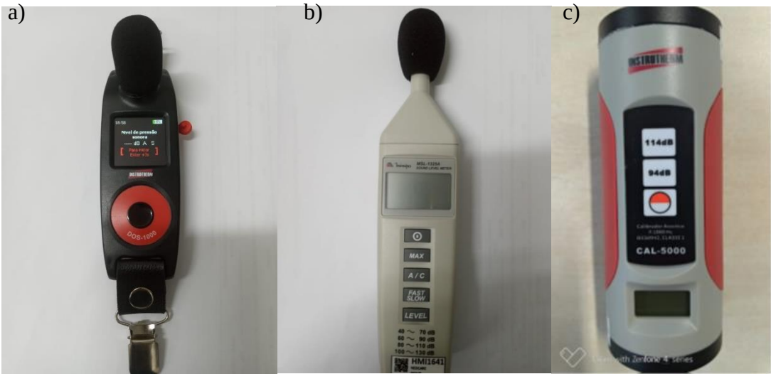
Figura 12– a) Modelo: DOS-1000. Instrumento de Medição de Pressão Sonora; b) MSL 1325A. Instrumento de Medição de Pressão Sonora; Fabricante: Mimipa , c) Calibrador; Fabricante: Instruterm; Modelo: CAL-5000
