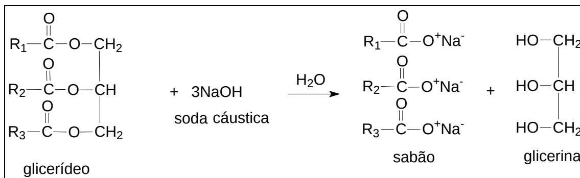
Figura 1- Reação que descreve o processo de saponificação
