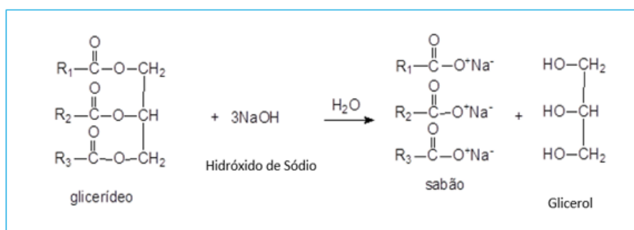
Figura 1 – Representação da reação de saponificação
