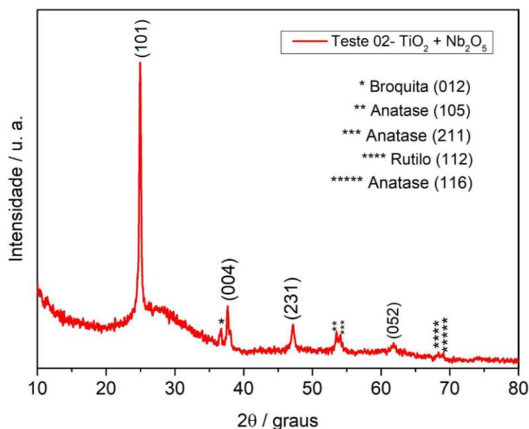
Figura 1 - Difratomogramas de raios X do catalisador híbrido de titânio e nióbio
