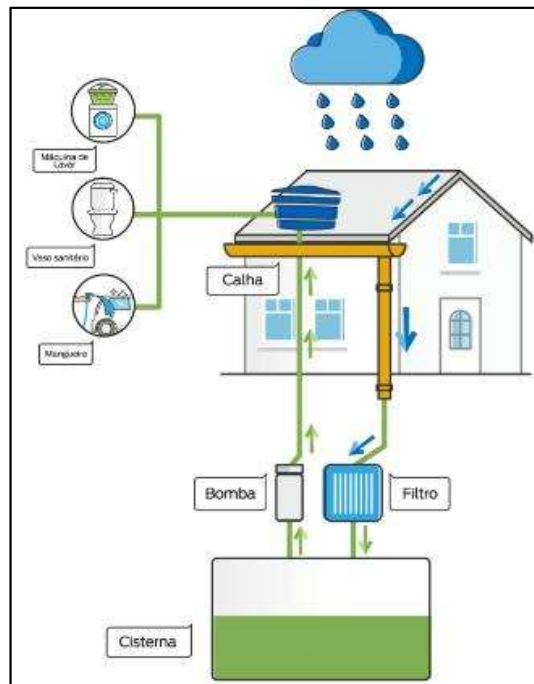
Figura 26 - Captação de água da chuva por calha
