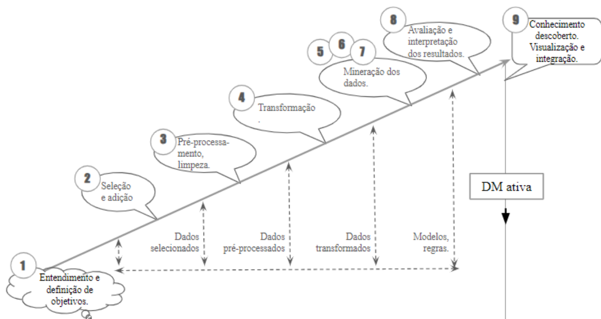
Figura 2 – O Processo de Knowledge Discovery em Bases de Dados
