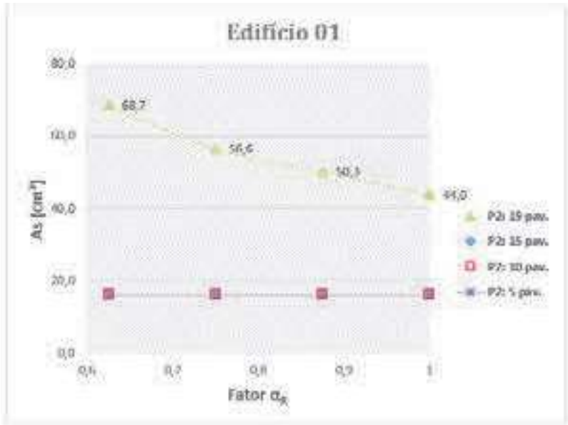
Figura 61 – Edifício 1: armadura do pilar P2 versus fator \alpha_R Fonte: Elaborada pela autora.
