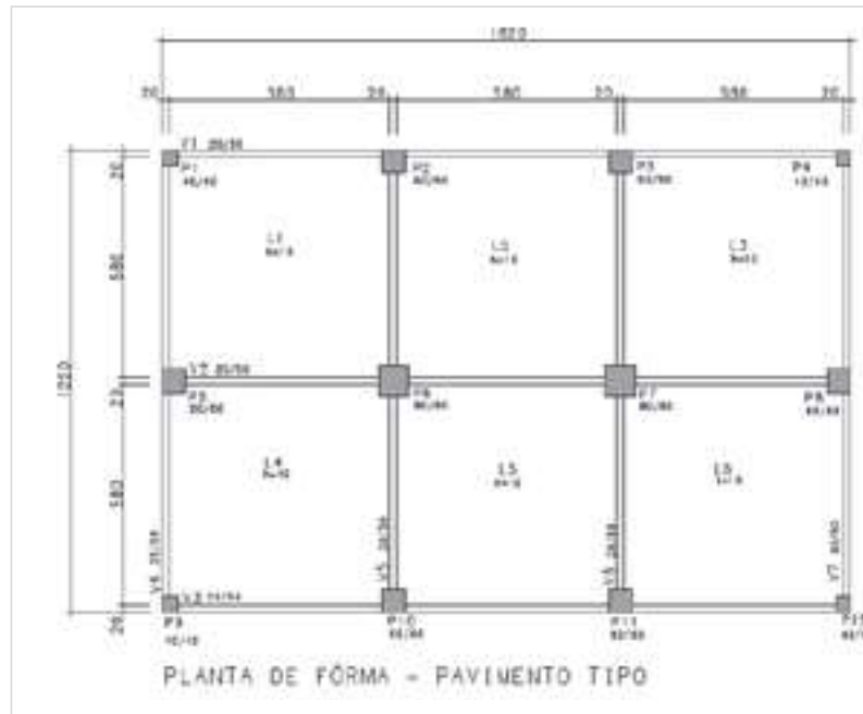
Figura 3 – Planta de formas do Edifício 1
