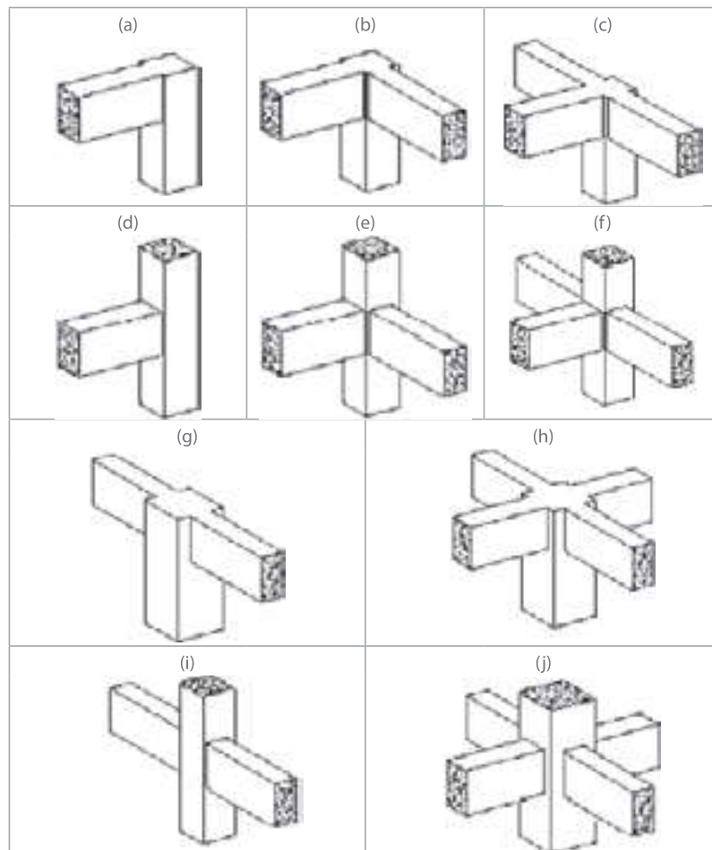
Figura 8 – Geometrias usuais de ligações viga-pilar
