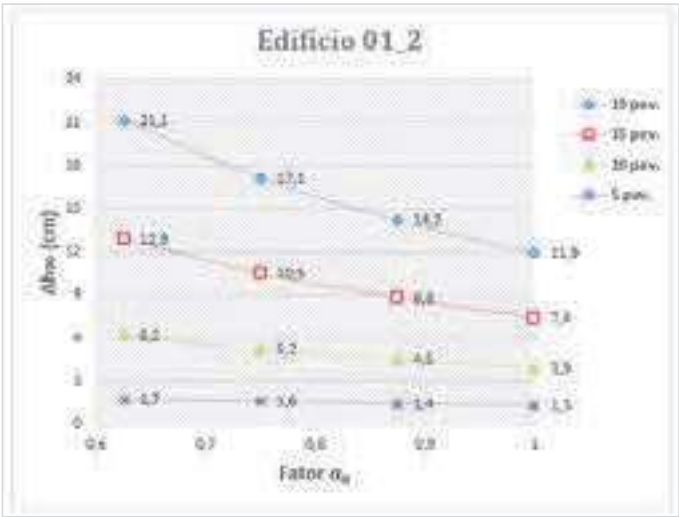
Figura 63 – Edifício 1_2: deslocamento horizontal no topo da estrutura versus fator \alpha_R Fonte: Elaborada pela autora.
