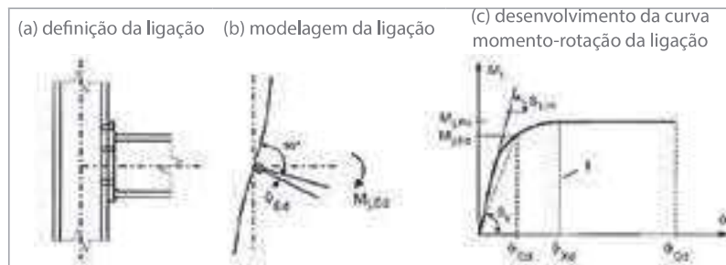
Figura 17 – Curva momento-rotacão para uma ligação viga-pilar
