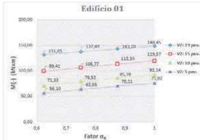
Figura 56 – Edifício 1: momento negativo da viga V2 versus fator \alpha_R
