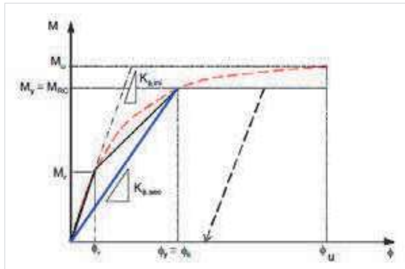
Figura 36 – Rigidez secante para a curva momento-rotação
