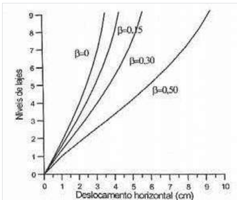
Figura 30 – Deslocamentos horizontais do pórtico de contraventamento para diferentes graus de flexibilidade dos nós
