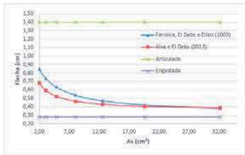
Figura 49 – Influência da armadura negativa na flecha
