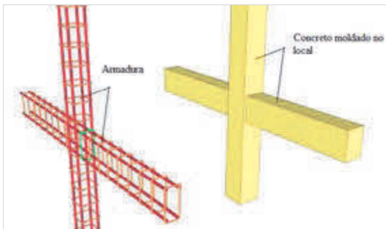
Figura 6 – Ligação viga-pilar em concreto armado moldado no local
