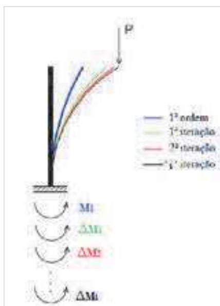
Figura 23 – Processo iterativo para determinação do momento fletor atuante na base da edificação
