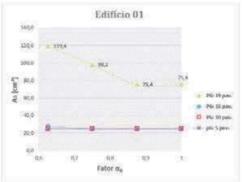
Figura 62 – Edifício 1: armadura do pilar P6 versus fator \alpha_R Fonte: Elaborada pela autora.
