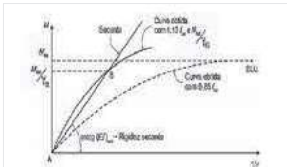
Figura 22 – Relação momento-curvatura
