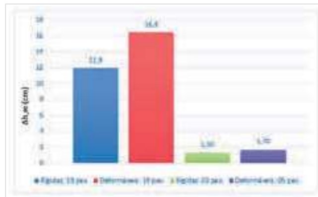
Figura 84 – Modelo de Ferreira, El Debs e Elliot (2003): deslocamento horizontal da estrutura com 19 e 5 pavimentos, considerando ligações rígidas e ligações deformáveis Fonte: Elaborada pela autora.
