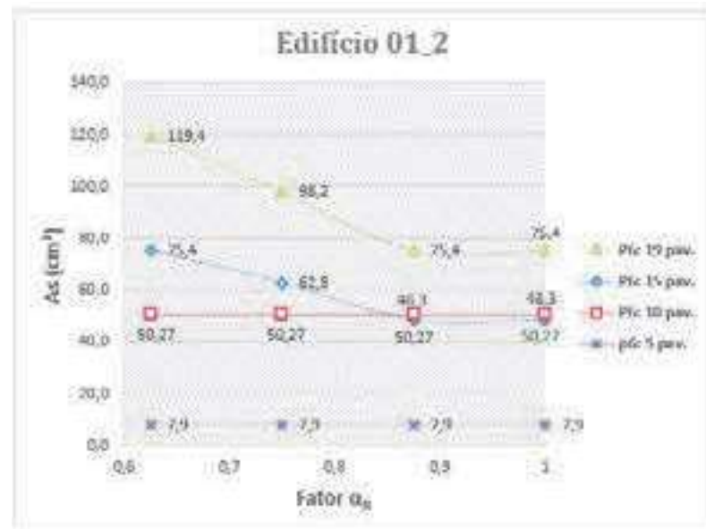
Figura 71 – Edifício 1_2: armadura do pilar P6 versus fator \alpha_R Fonte: Elaborada pela autora.
