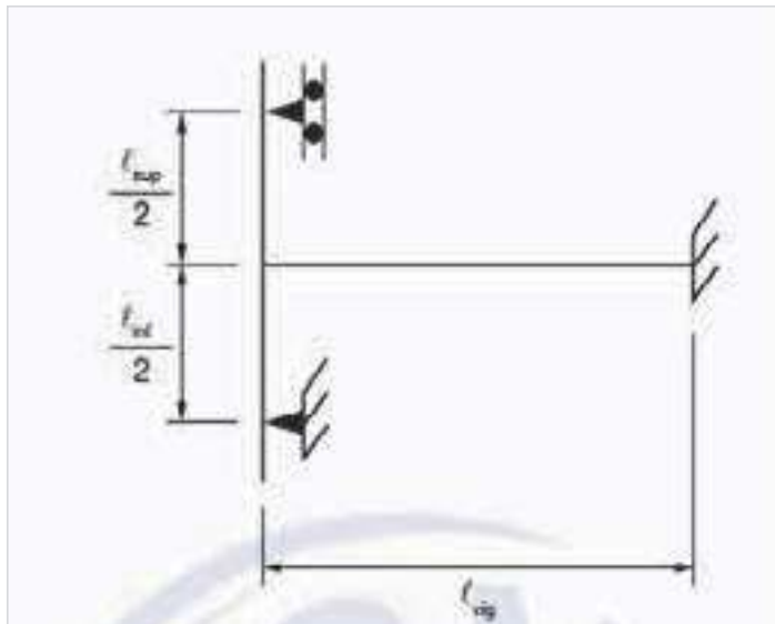
Figura 19 – Aproximação permitida em apoios extremos
