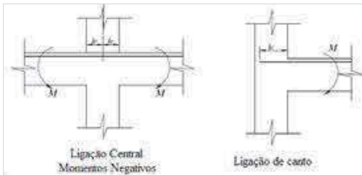
Figura 38 – Comprimento de embutimento para ligações viga-pilar monolíticas
