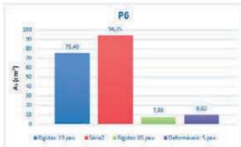
Figura 90 – Modelo de Ferreira, El Debs e Elliot (2003): armadura do pilar P3 da estrutura com 19 e 5 pavimentos, considerando ligações rígidas e ligações deformáveis Fonte: Elaborada pela autora.
