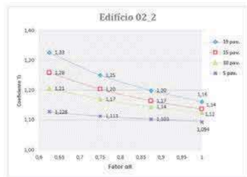
Figura 75 – Edifício 2_2: coeficiente \gamma_z versus fator \alpha_R Fonte: Elaborada pela autora.
