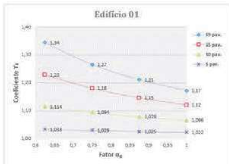
Figura 55 – Edifício 1: coeficiente \gamma_z versus fator \alpha_R
