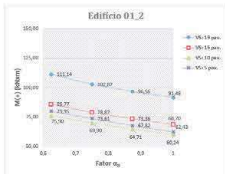
Figura 68 – Edifício 1_2: momento positivo da viga V5 versus fator \alpha_R Fonte: Elaborada pela autora.
