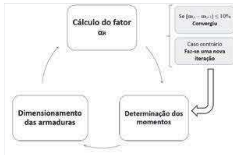
Figura 76 – Processo iterativo para determinação do fator \alpha_R das ligações Fonte: Elaborada pela autora.
